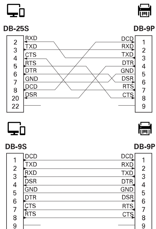
Рисунок 15 Подключение принтера к устройству DCE
