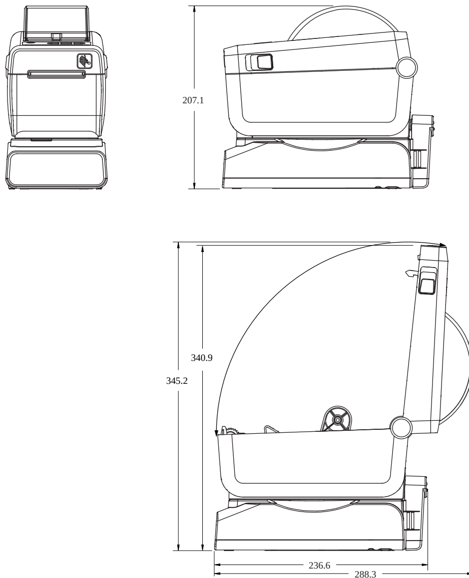
Рисунок 19 Принтер ZD411D с дополнительным модулем присоединяемой аккумуляторной базовой станции (размеры в миллиметрах)
