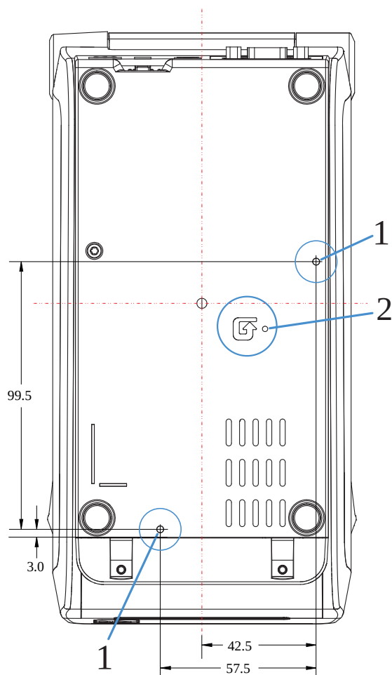
Рисунок 20 Стандартный монтаж ZD411D (размеры в миллиметрах)
