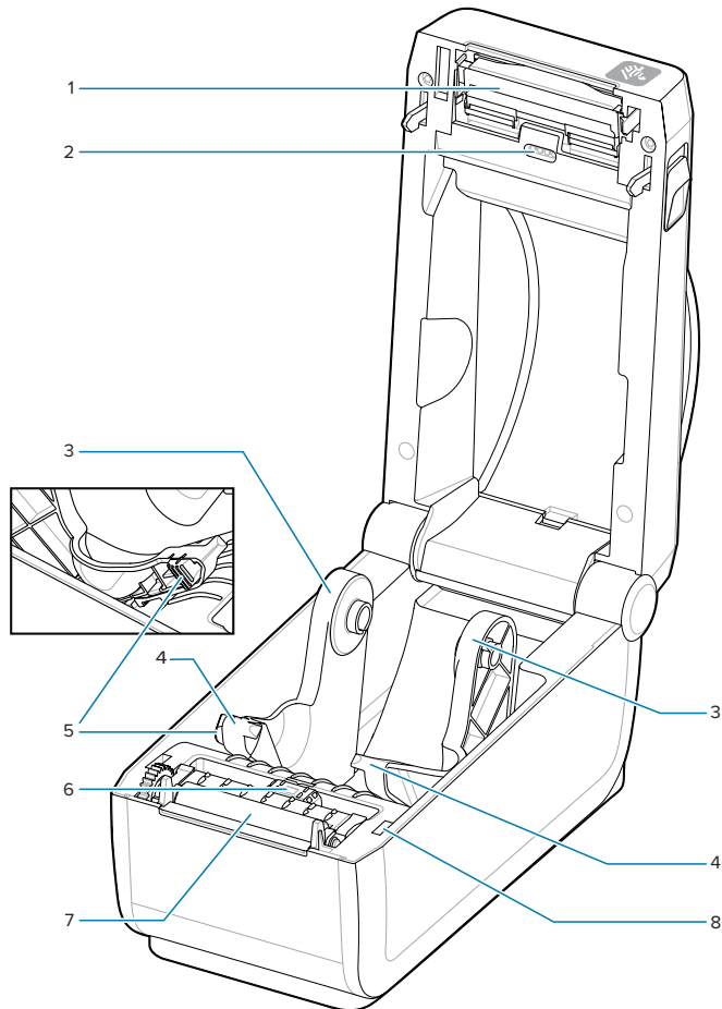
Рисунок 3 Внутренние компоненты принтера
