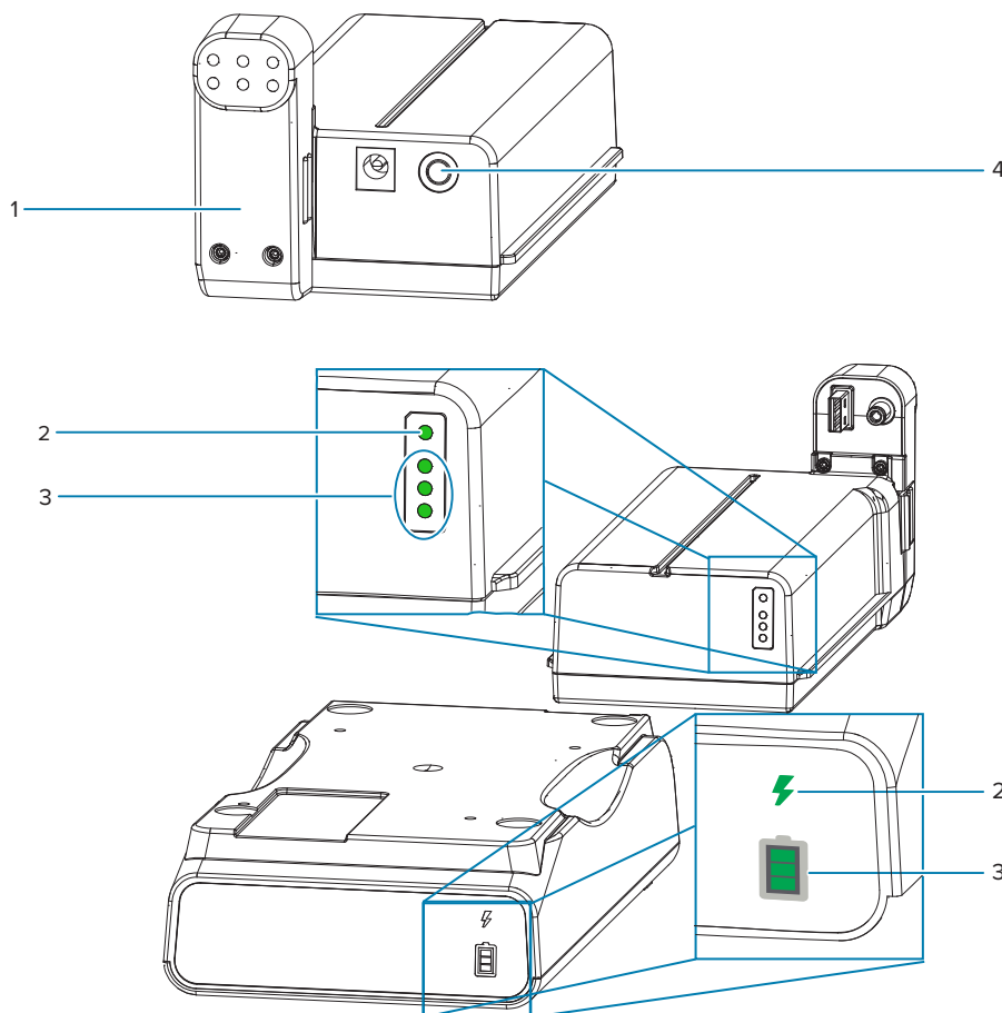
Рисунок 6 Элементы управления аккумулятора
