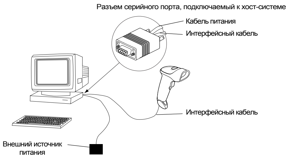
Рисунок 6-1 Прямое подключение посредством интерфейса RS-232
