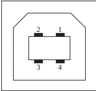
Рисунок 14 USB-B
