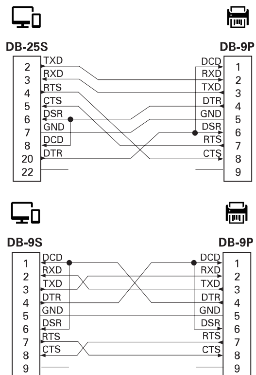
Рисунок 15 Подключение принтера к устройству DTE
