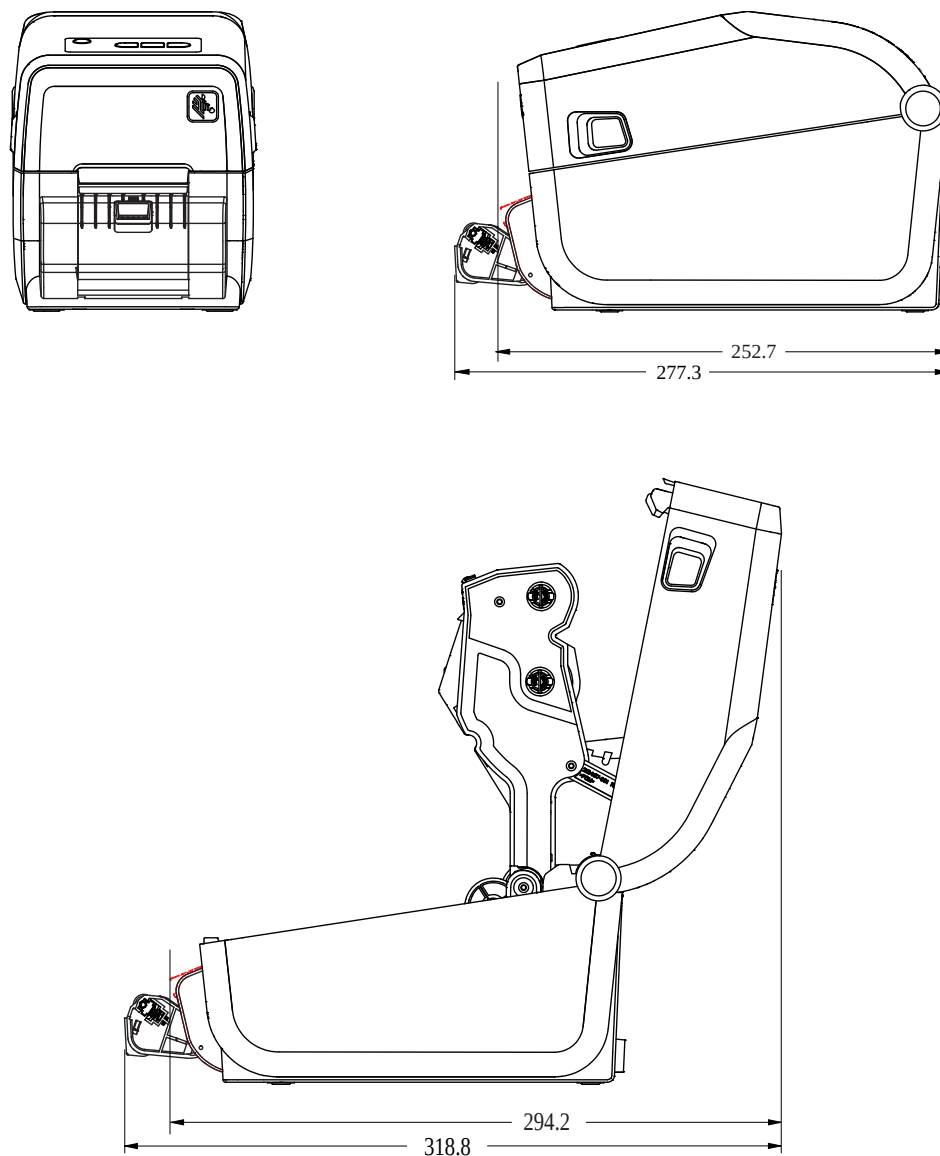
Рисунок 18 Принтер ZD411T с дополнительным модулем для этикеток (размеры в миллиметрах)
