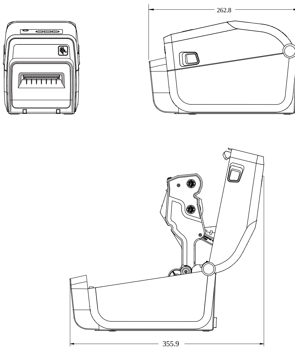
Рисунок 19 Принтер ZD411T с дополнительным модулем резака носителя (размеры в миллиметрах)
