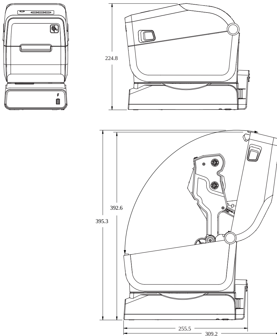
Рисунок 20 Принтер ZD411T с дополнительным модулем присоединяемой аккумуляторной базовой станции (размеры в миллиметрах)
